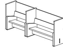
Sitzbank L Föhre L: 3.7 m B: 0.8 m H: 1.4 m
